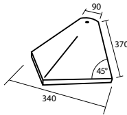
A000 3400 * Arêtier fermé pour 16 x 27 (10,0 au ml)
