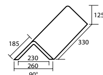
A000 1800* Faîtière angulaire 90° (3,0 au ml)
