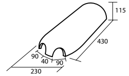
A000 5880 Rencontre faitière demi-ronde 2 pans
