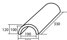
A000 1400 Faîtière demi-ronde (3,0 au ml)
