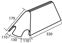
A000 5800 * Rencontre faitière angulaire 2 pans
