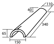
A000 3800* Arêtier de chevauchement "tige de botte" (3,5 au ml)
